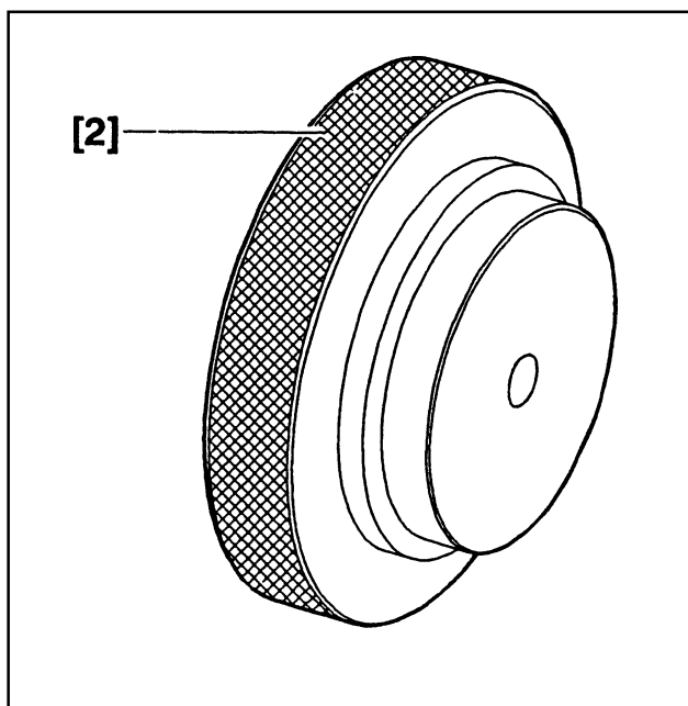
[2] Оправка для установки маслоотражающего уплотнения левого приводного вала (-).0342 С
