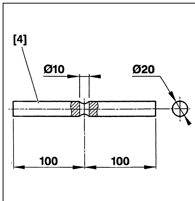
[4] Приспособление для демонтажа входного вала (этот инструмент должен быть изготовлен из стали в ремонтном цехе)
