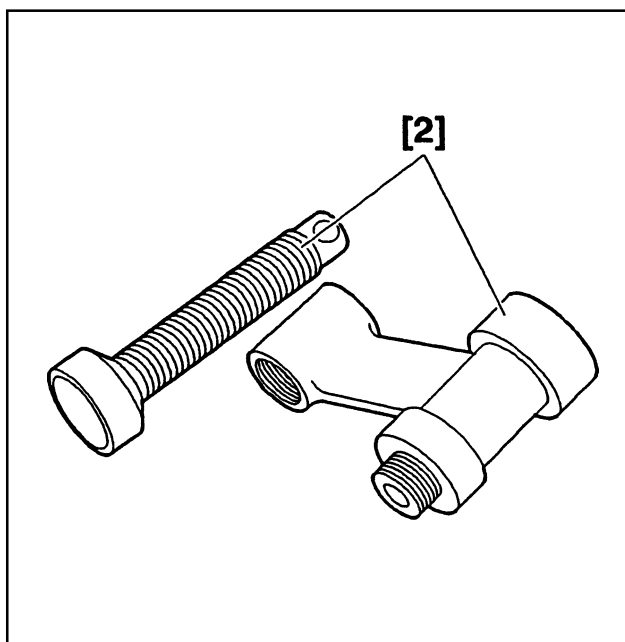
[2] Приспособление для демонтажа и установки стопорных колец тормоза F2 (-).0342 Q
