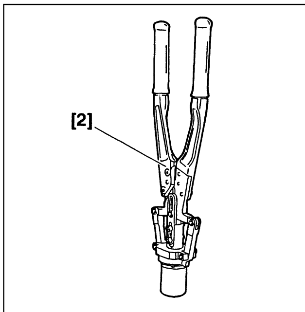
[2] Приспособление для установки гайки планетарного ряда (-).0342 P
