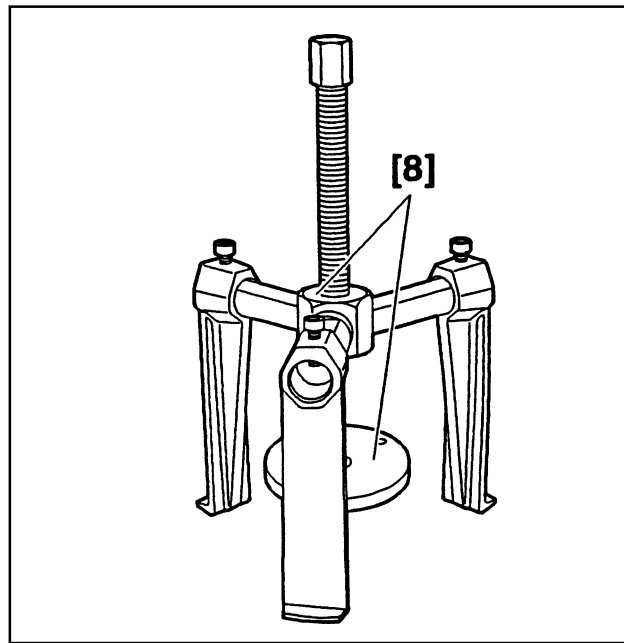
[8] Съемник большого подшипника дифференциала (-).0342 A
