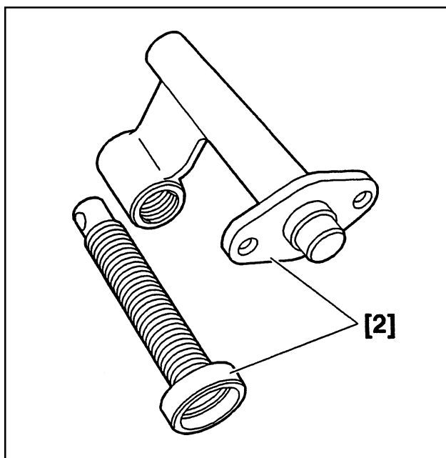
[2] Приспособление для демонтажа и установки стопорных колец тормоза F3 (-).0342 R
