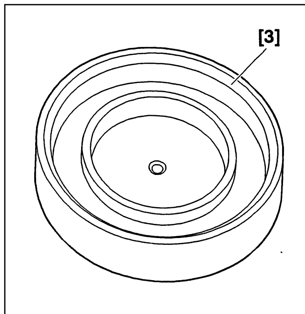
[3] Приспособление для придания предварительной формы кольцевому поршню фрикциона E1 (-).0342 AB
