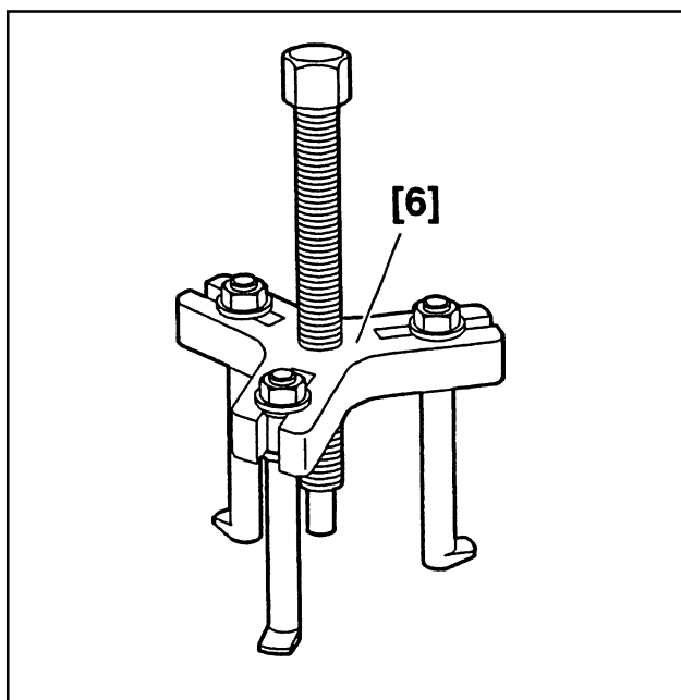
[6] Съемник сепаратора большого подшипника дифференциала (-).0342 M
