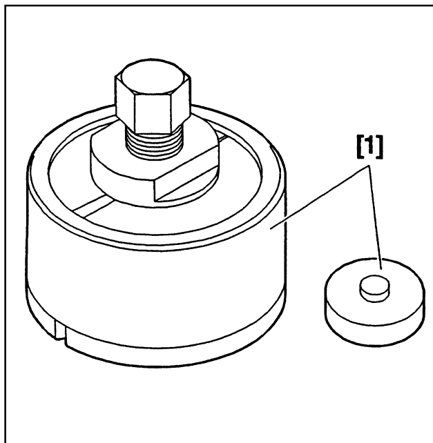
[1] Съемник подшипников второго планетарного ряда (-).0342 К
