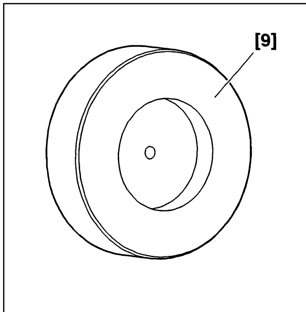
[9] Оправка для установки сепаратора большого подшипника дифференциала (-).0342 AL
