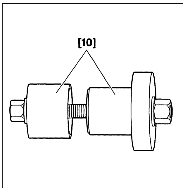
[10] Оправка для установки большого подшипника дифференциала (-).0342 Н
