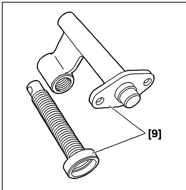
[9] Приспособление для демонтажа и установки стопорных колец тормоза F3 (-).0342 R
