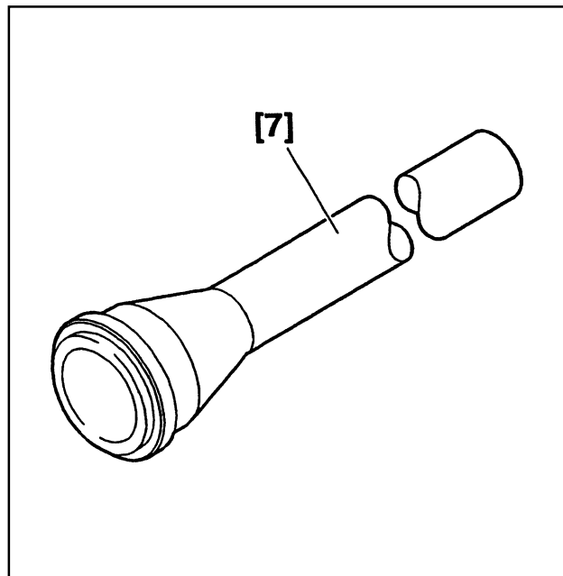
[7] Пробойник для установки уплотнения левого приводного вала (-).0338 H1
