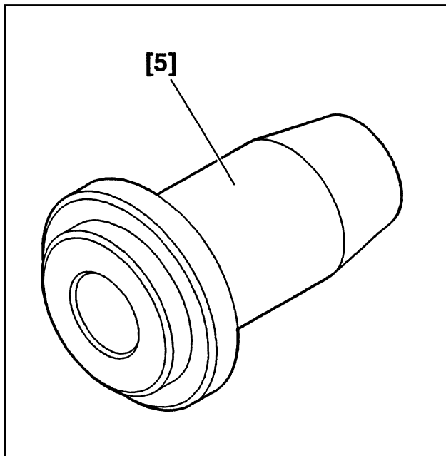
[5] Пробойник для установки уплотнения правого приводного вала (-).0338 J1
