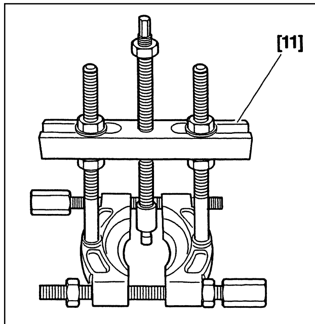
[11] Съемник малого подшипника дифференциала 4108-Т
