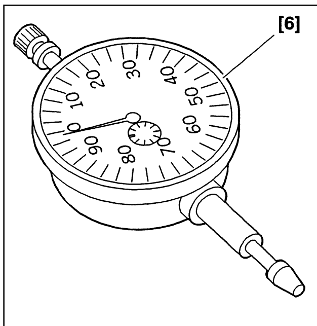
[6] индикаторная головка для измерения зазора (-).0337 Н
