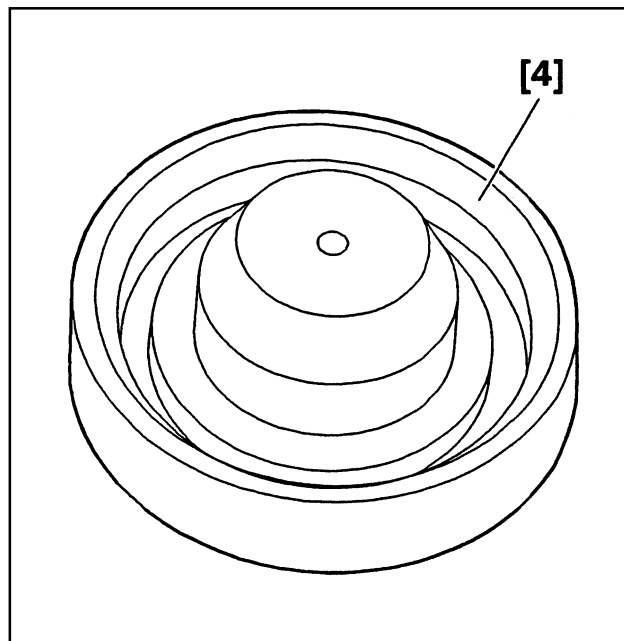
[4] Приспособление для придания предварительной формы поршню фрикциона E1 (-).0342 AC
