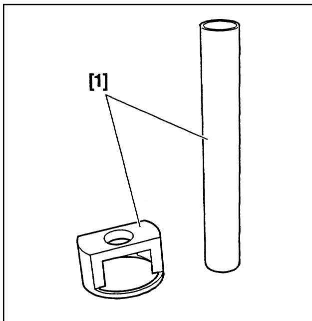
[1] Съемник кольцевого поршня фрикциона E2 (-).0342 AE
