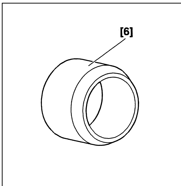
[6] Оправка для установки поршня фрикциона E2 (-).0342 AG
